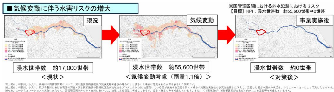
図4-15 利根川下流部における気候変動に伴う水害リスク
