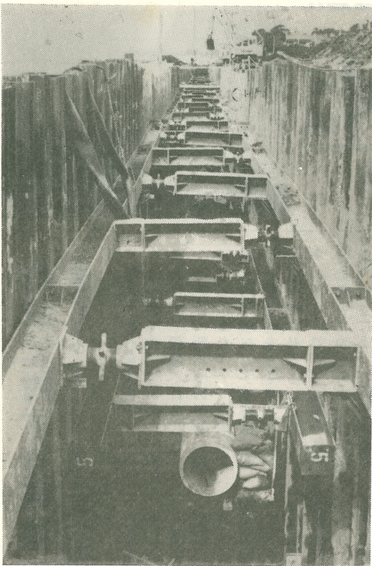
▲利根町公共下水道建設に伴う第一汚水幹線埋設工事。 2月28日羽中地先にて撮影。 早期完成が望まれています。
