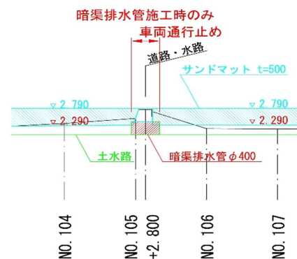
縦断図 V=1:100 H=1:1000
